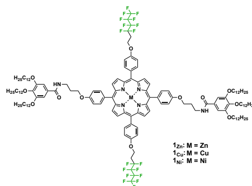
図1 モノマー分子の構造
