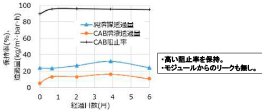
図: 6ヶ月膜分離試験結果
