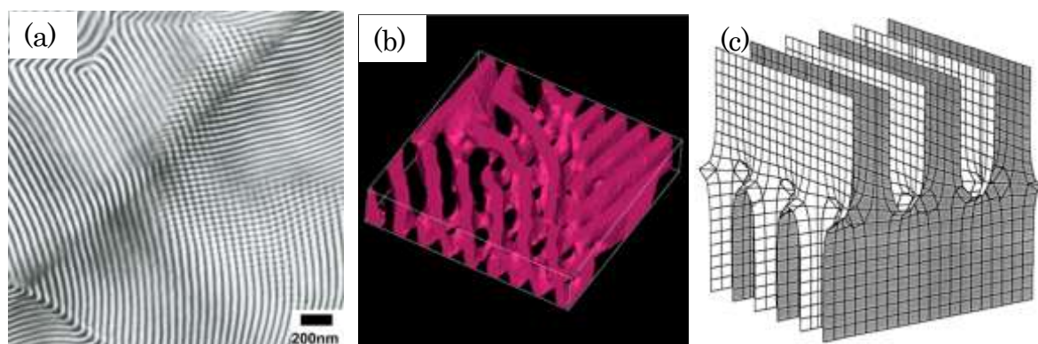
Figure 9 (a) PS- b -PI(1)単体に見られるラメラグレインバウンダリーのTEM像 (b) ラメラグレインバウンダリーの3D-TEM像 (c) SHERK's surface モデル
