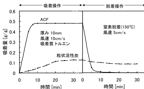
図8 ACFと粒状活性炭の脱着特性
