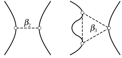
図 2. 線状鎖の A_2 における \beta_2 と \beta_3
