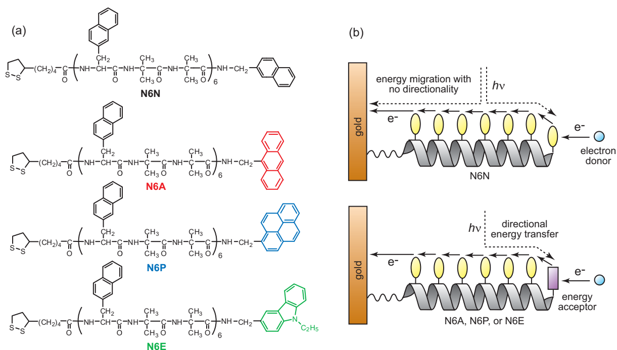
図9 末端に光エネルギーアクセプターを結合したヘリックスペプチド。ナフチル基が吸収した光エネルギーが効率良く光アクセプターに移動することで、水溶液中の電子ドナーによる還元反応を促進し、量子効率を向上させることを目指した。 4)
