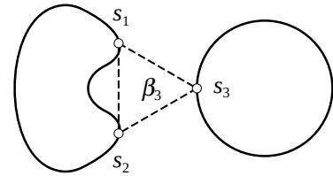
図 4. 環状鎖の A_2 における \beta_3
