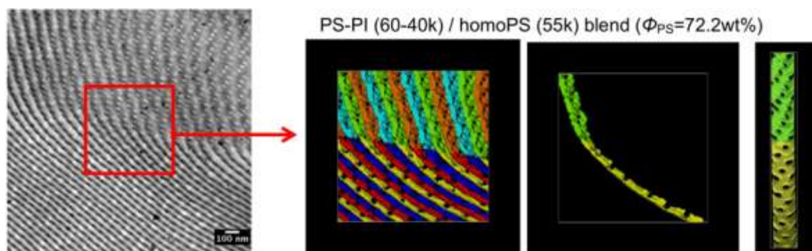
Figure 7 PS- b -PI(1)/ hPS(1) \phi_{PS} = 0.722 ブレンドの PL/PL 鈍角グレインバウンダリーの 2D-TEM および 3D-TEM イメージ、および 1 枚の PL 層の観察。
