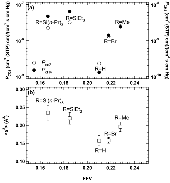
図 3 (a) FFV と P_{CO_2} 及び P_{CH_4} との関係。 (b) FFV と \langle u^2 \rangle との関係。
