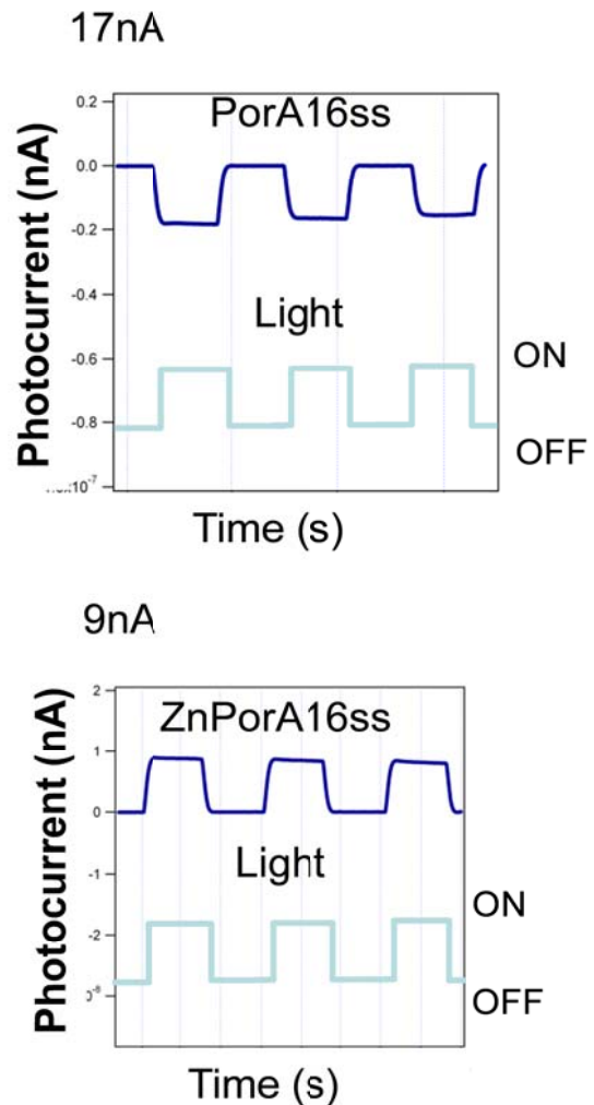
図7 ポルフィリンとポルフィリン亜鉛錯体とをN末端に導入したヘリックスペプチドでの光電流発生。
