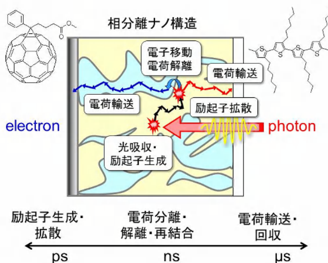
Figure 1 高分子薄膜太陽電池 (BHJ 型素子) における相分離ナノ構造と、その内部で起こる光電変換の素過程
