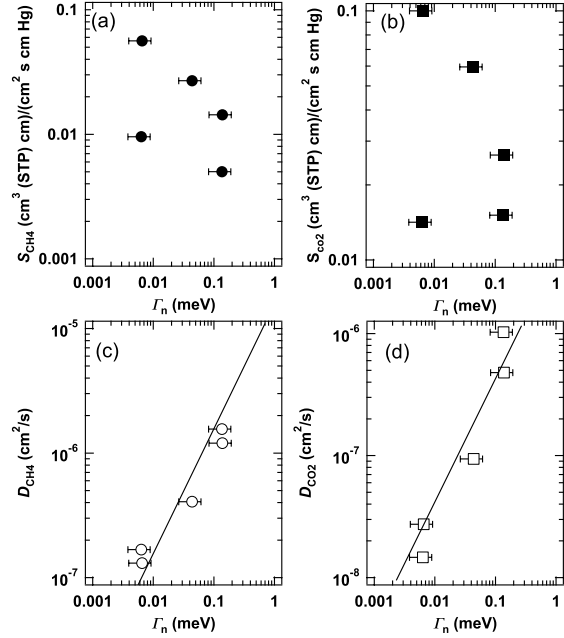
図 9 (a) S_{CH_4} と \Gamma_n との相関。(b) S_{CO_2} と \Gamma_n との相関。(c) D_{CH_4} と \Gamma_n との相関。(d) D_{CO_2} と \Gamma_n との相関。
