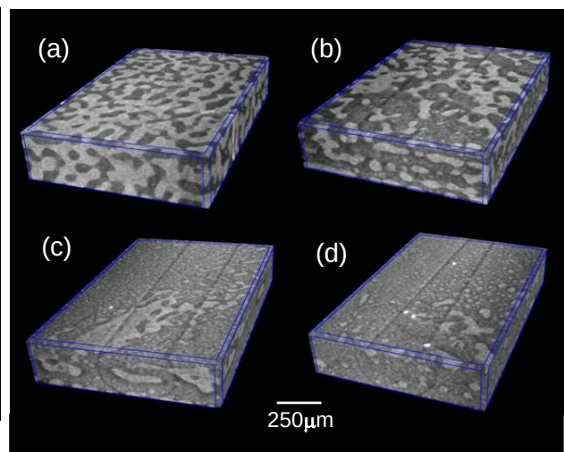
図 10 PS/PC ブレンドの X 線 CT 画像
