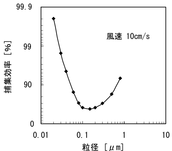
図 11 繊維層フィルターの粒径別捕集効率
