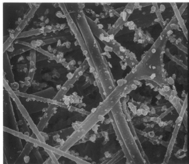
図 12 濾過後の繊維層フィルターの SEM 写真
