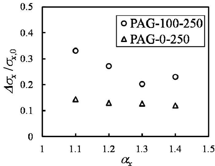
図4 高分子電解質ゲルおよび電氣的に中性の高分子ゲルの応力の相対減少量（ \Delta\sigma_x / \sigma_{x,0} ）の伸長比（ \alpha_x ）依存性
