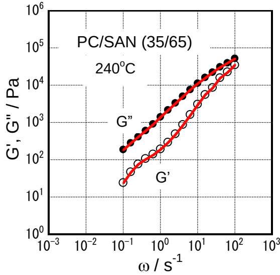
図 13 PC/SAN の動的粘弾性関数と Palierne 理論の予測値
