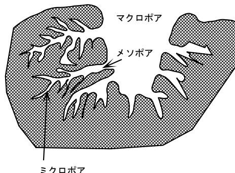
図3 粒状活性炭の細孔構造
